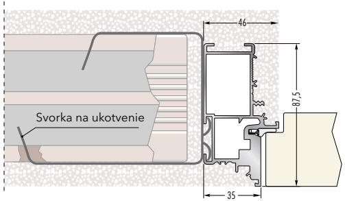
Zárubňa pre murovanú stenu s omietkou
