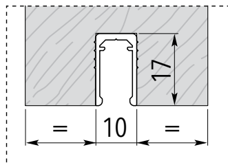
Detail dverného krídla s ochranným profilom
