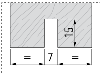
Detail dverného krídla s vyfrézovanou drážkou, ak ochranný profil nebude použitý
